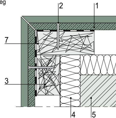
1C Részletrajz – Külső sarok kialakítása gérbévágással
