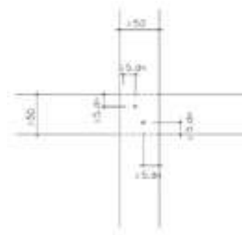
keresztpontonként 2 rögzítőelem
