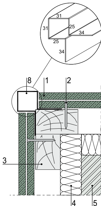
1A Részletrajz – Külső sarok kialakítása színes alumínium profillal
