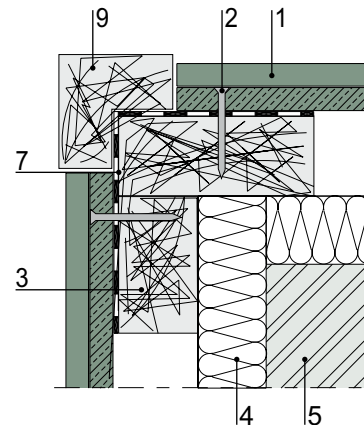
1C Részletrajz – Külső sarok kialakítása gérbévágással
