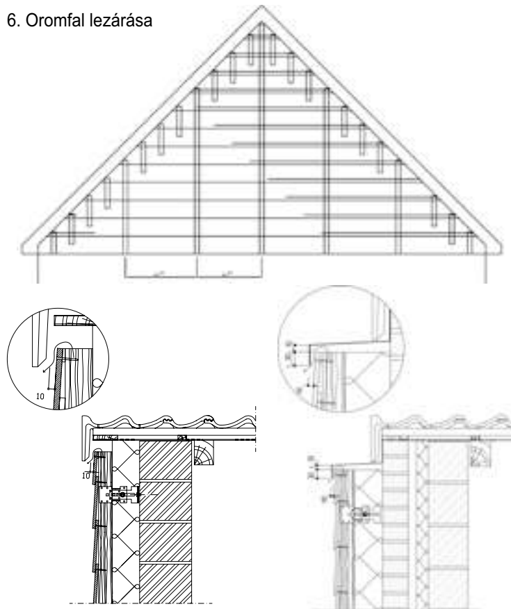
6A Részletrajz - új építésű homlokzatburkolat csatlakoztatása az oromszegélyhez
